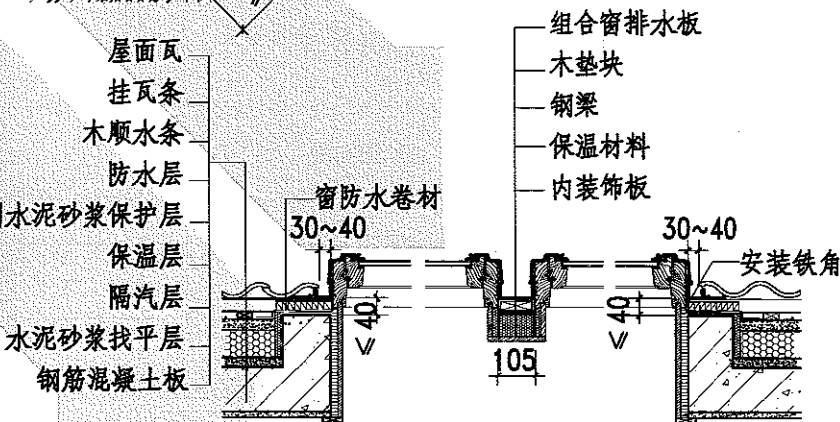
水平剖面
