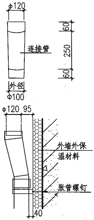
② 水落管接口
