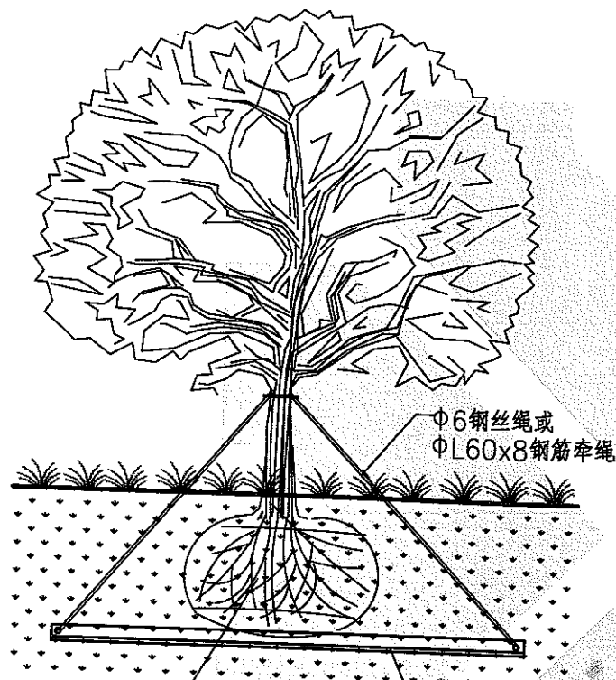
剖面示意
