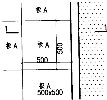
① 架空板凳步道局部平面 (土层厚度 ≤ 400)
