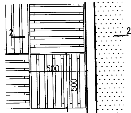
② 木格板步道局部平面 (土层厚度 ≤ 300)
