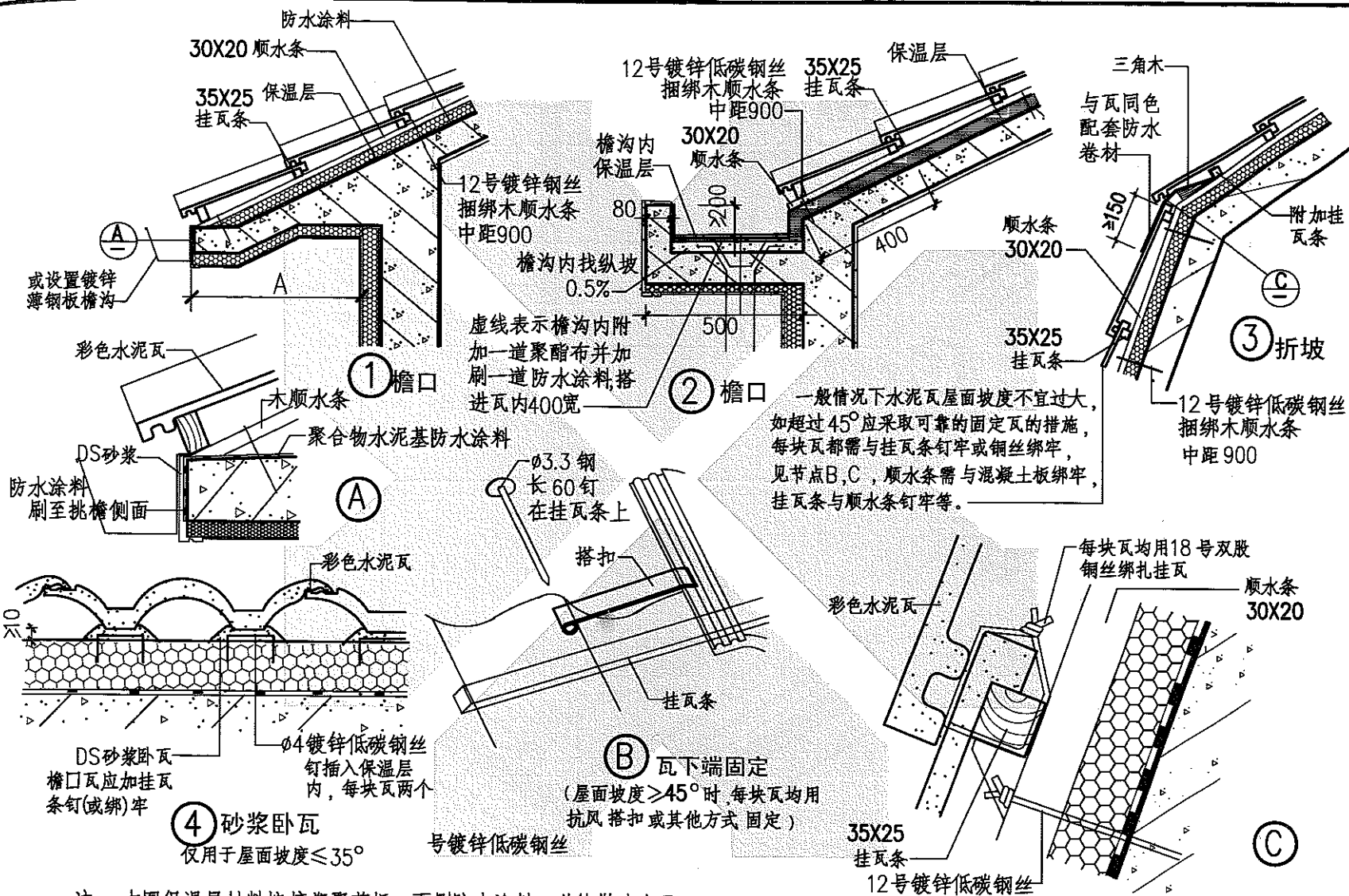
图名 彩色水泥瓦屋面详图(1)
