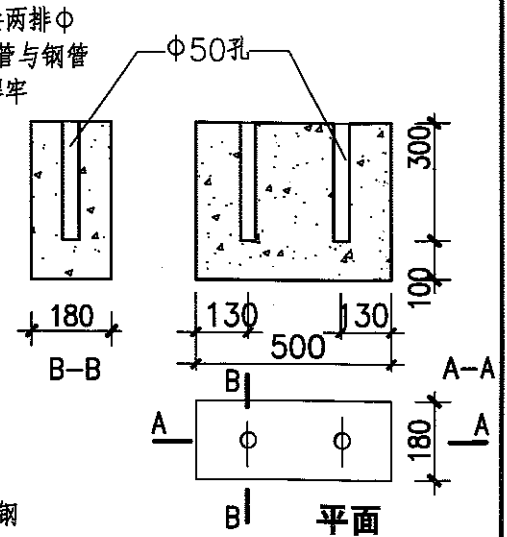
预制混凝土底座
