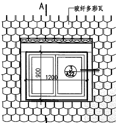
① 单个老虎窗立面
