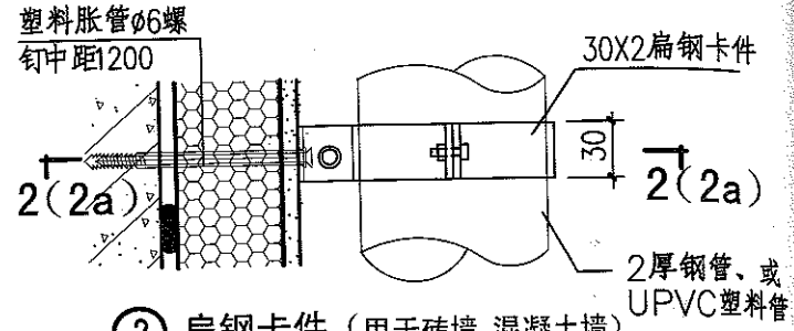
② 扁钢卡件 (用于砖墙、混凝土墙)
