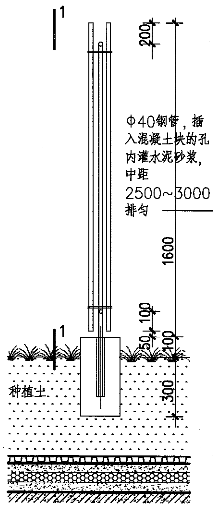
① 竹围栏剖面 竹围栏适用于户与户之间绿化的分隔, 靠竹围栏处可种植爬藤, 形成绿篱。
