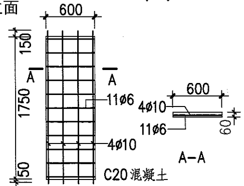
预制混凝土檐口板
