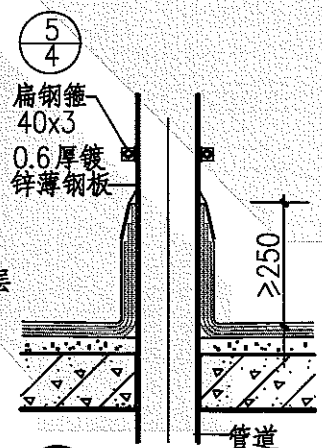
④ 管道出屋面处
