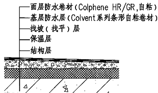
④ 混凝土屋面条粘防水系统
