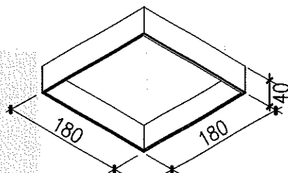
① 通风口盖 2厚镀锌薄钢板制作
