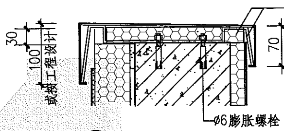
② 女儿墙铝板压顶
