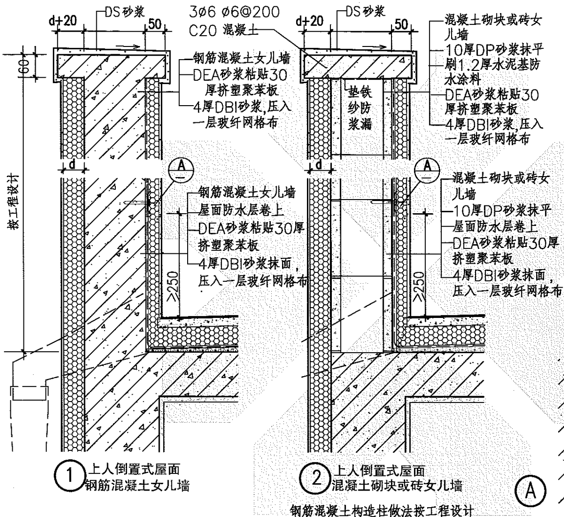
图名 倒置式上人屋面女儿墙详图
