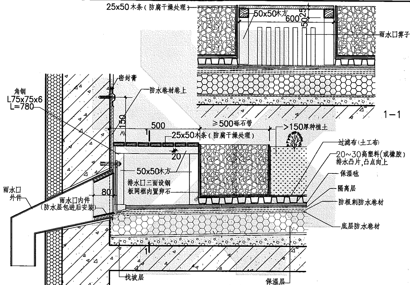
① 外排水口处详图
