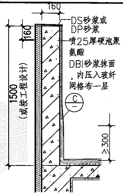
② 钢筋混凝土女儿墙 (上人屋面)
