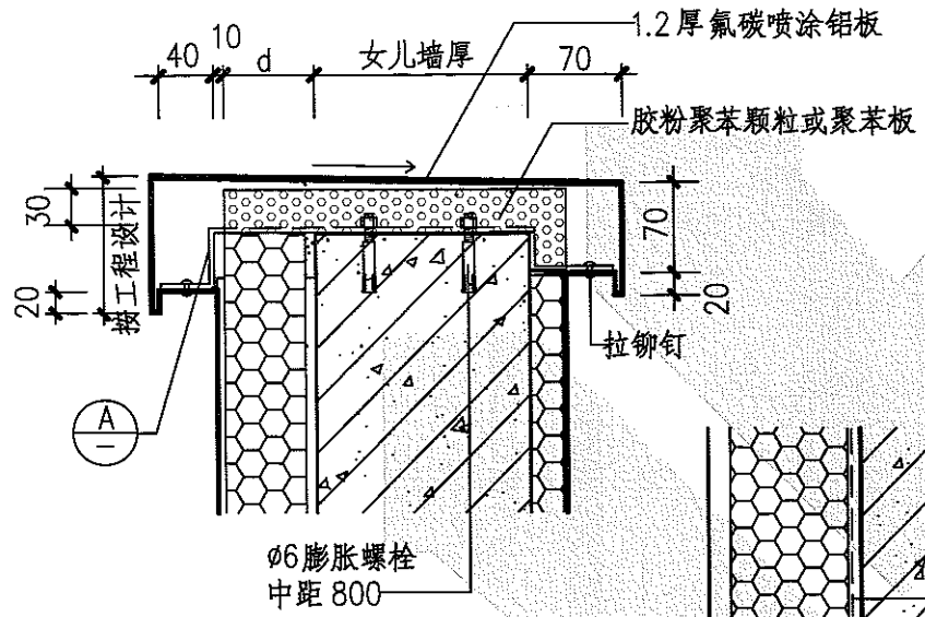
① 女儿墙铝板压顶
