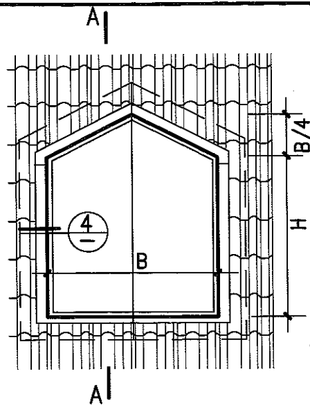
老虎窗立面
