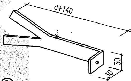
②埋件 30X3扁钢
