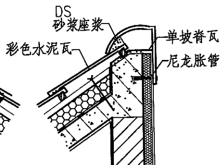
② 单坡屋脊
