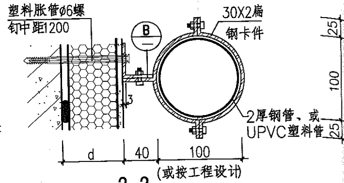
② 扁钢卡件 (用于砖墙、混凝土墙)
