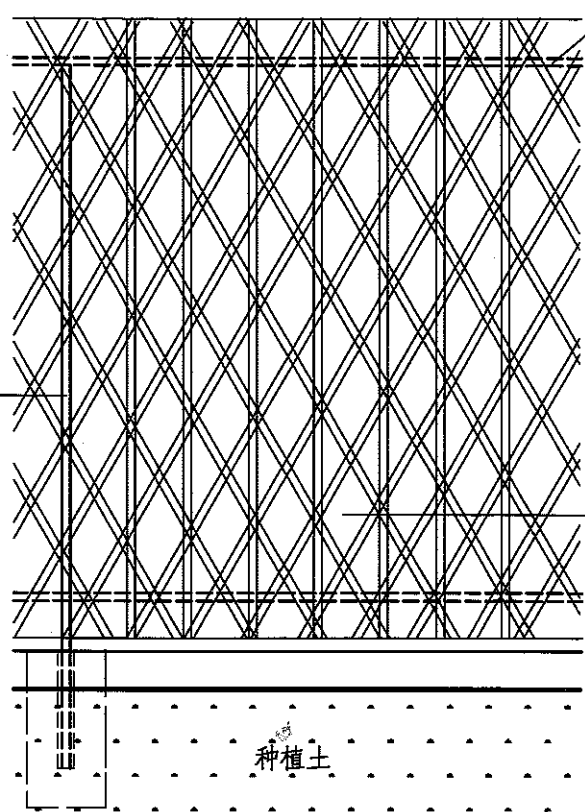
1-1 竹篱立面
