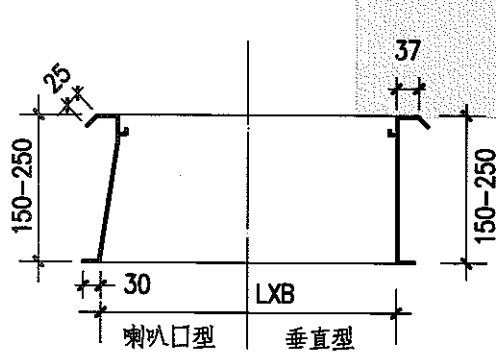
大型混凝土预制板结构采光口组合示意
