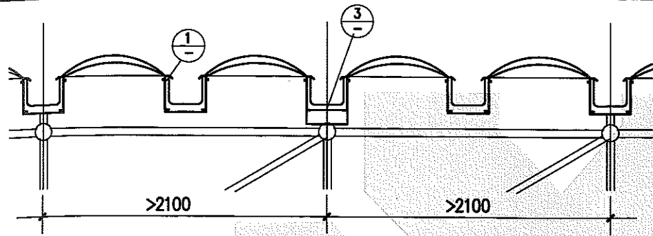
网架结构采光口组合示意
