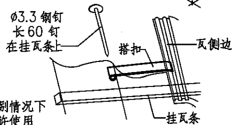
瓦下端 (屋面坡度 \geq 35^\circ 时,每块瓦均用搭扣或其他方式固定)
