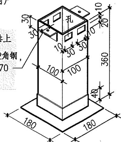
② 2厚镀锌薄钢板制作
