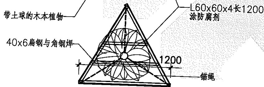
土中三角形埋件平面
