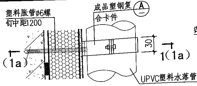
① 塑钢复合卡件 (用于砖墙、混凝土墙)
