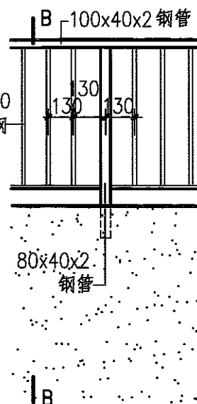
2 立面示意
