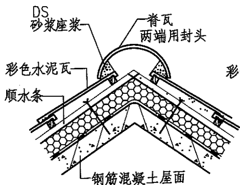
① 屋脊
