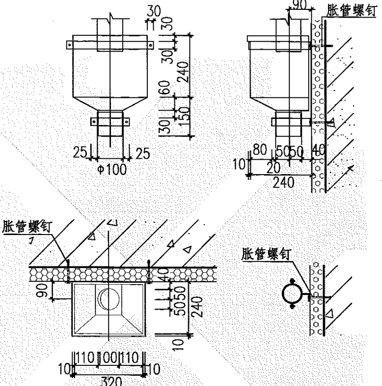
① 钢板水斗平面
