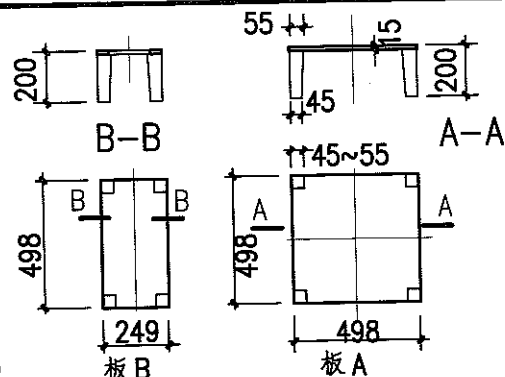
纤维水泥架空板凳平面 板A 500x500, 板B 250x500, 根据步道宽度选用。
