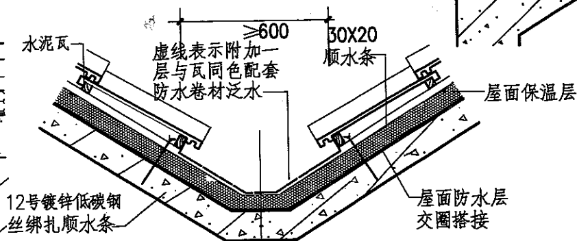
⑥ 天沟
