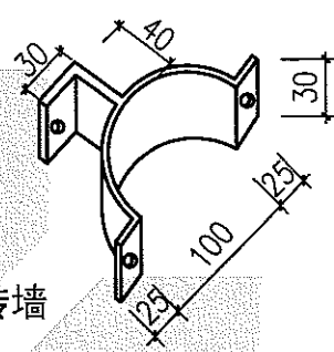
①成品塑钢复合卡件或30X2扁钢卡子
