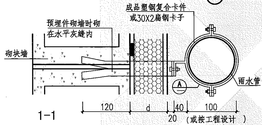
①用于砌块墙 空心砖墙
