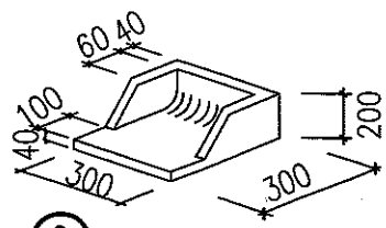
③ 水簸箕
