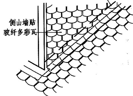
老虎窗侧面与屋面关系
