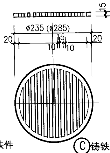
图名 直式雨水口 (1)
