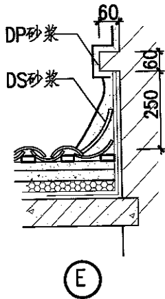
高出屋面墙体与屋面泛水
