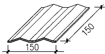
波纹装饰瓦示意 陶质装饰瓦, 铺贴时用 高粘结强度胶配水泥砂 浆离年, 上下搭接10
