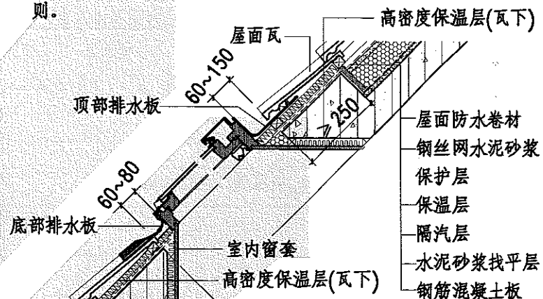
垂直剖面
