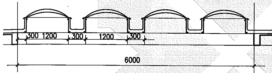
大型混凝土预制板结构采光口组合示意
