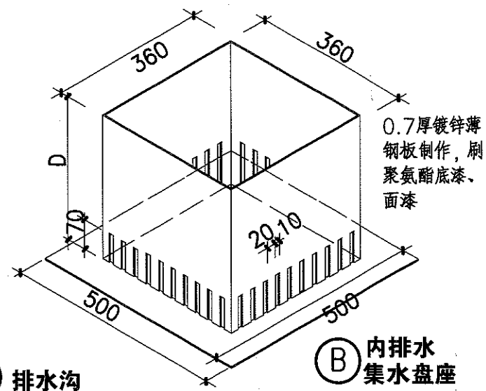
图名 内排水口详图
