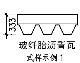
玻纤胎沥青瓦 式样示例1 用直径3的专用 钢钉固定
