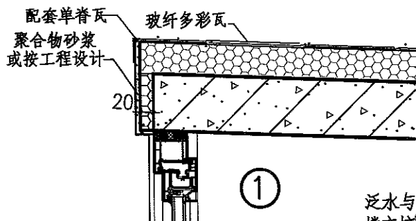
住宅坡屋面屋脊老虎窗构造示例
