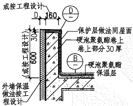
① 钢筋混凝土女儿墙 (不上人屋面)
