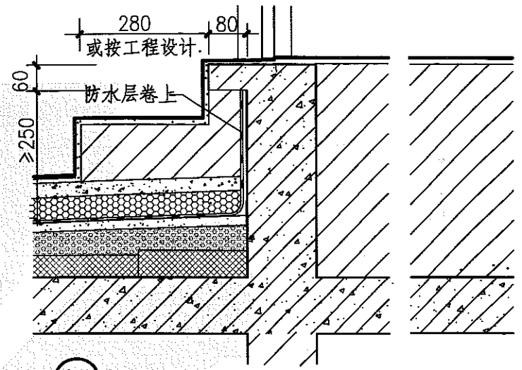
①a 倒置式屋面(门口无变形缝)
