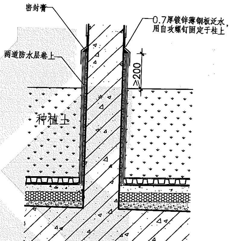
花架柱脚详图 (花架钢筋混凝土柱与钢筋混凝土屋面板连接)
